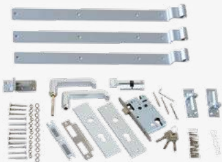
Universeel deurbeslag 006624 | € 85,- met deurbeslag, cilindslot, hang- en sluitwerk. Voor alle houten tuindeuren
